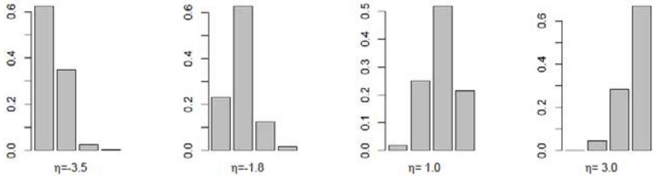
Ilustración 40. Función de probabilidad de masa de la distribución logística ordenada para diferentes valores de \eta , con \beta = (-3.0, 0.0, 2.3) , y K = 4 .
